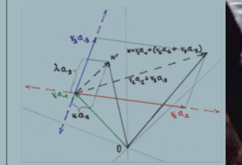
Bild 10: a' = v_1 a_1 + v_2 a_2 + v_3 a_3 Ebene, die nicht durch den Ursprung geht
